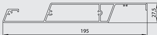
Průřez lamely
