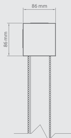
Rozměry kazety
