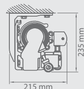
Stropní montáž
