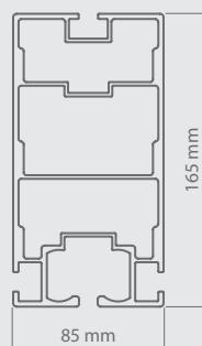
Průřez Vodící lišty
