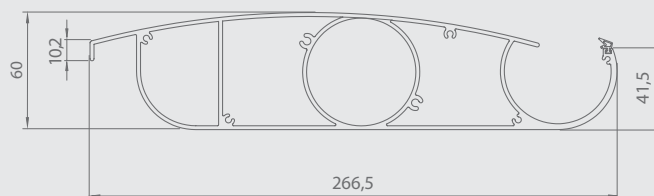
Průřez sloupu
