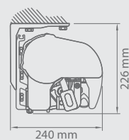
Stropní montáž
