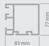
Průřez vodící lišty
