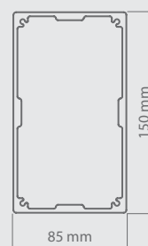
Průřez sloupu
