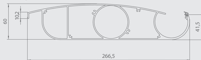
Průřez lamely
